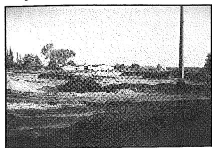
Het overstort ter hoogte van de Dregel. Bij hevige regenval moet het overtollige water in de riolen tijdelijk kunnen opgevangen worden. Aanvallig was het de bedoeling hiervoor de Dorpsloop te gebruiken. Omdat deze waterloop echter te klein is, moest er naar een alternatief gezocht worden. De aanplanting van riet in het overstort zal voor een biologische zuivering zorgen.
