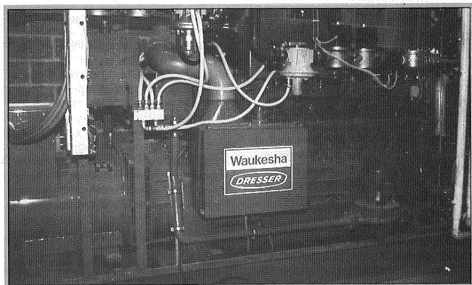
Deze gasmotor is gekoppeld aan een generator. Hij zet bio-gas om tot elektriciteit
