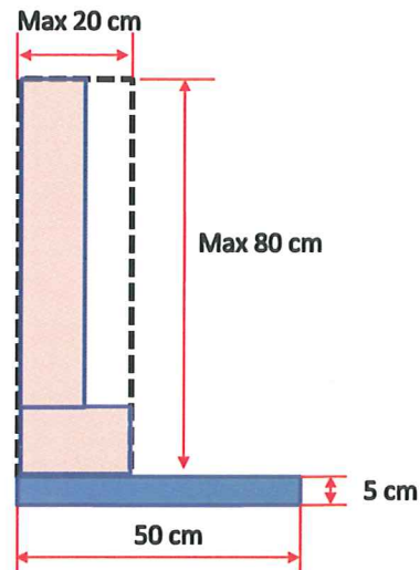
Zij aanzicht
