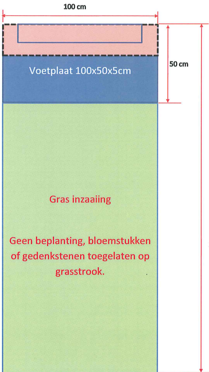
Boven aanzicht
